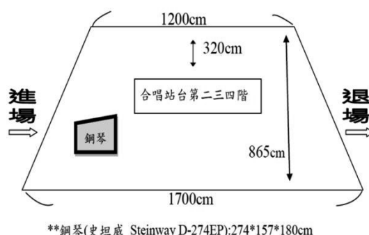
合唱舞台規格示意圖：
